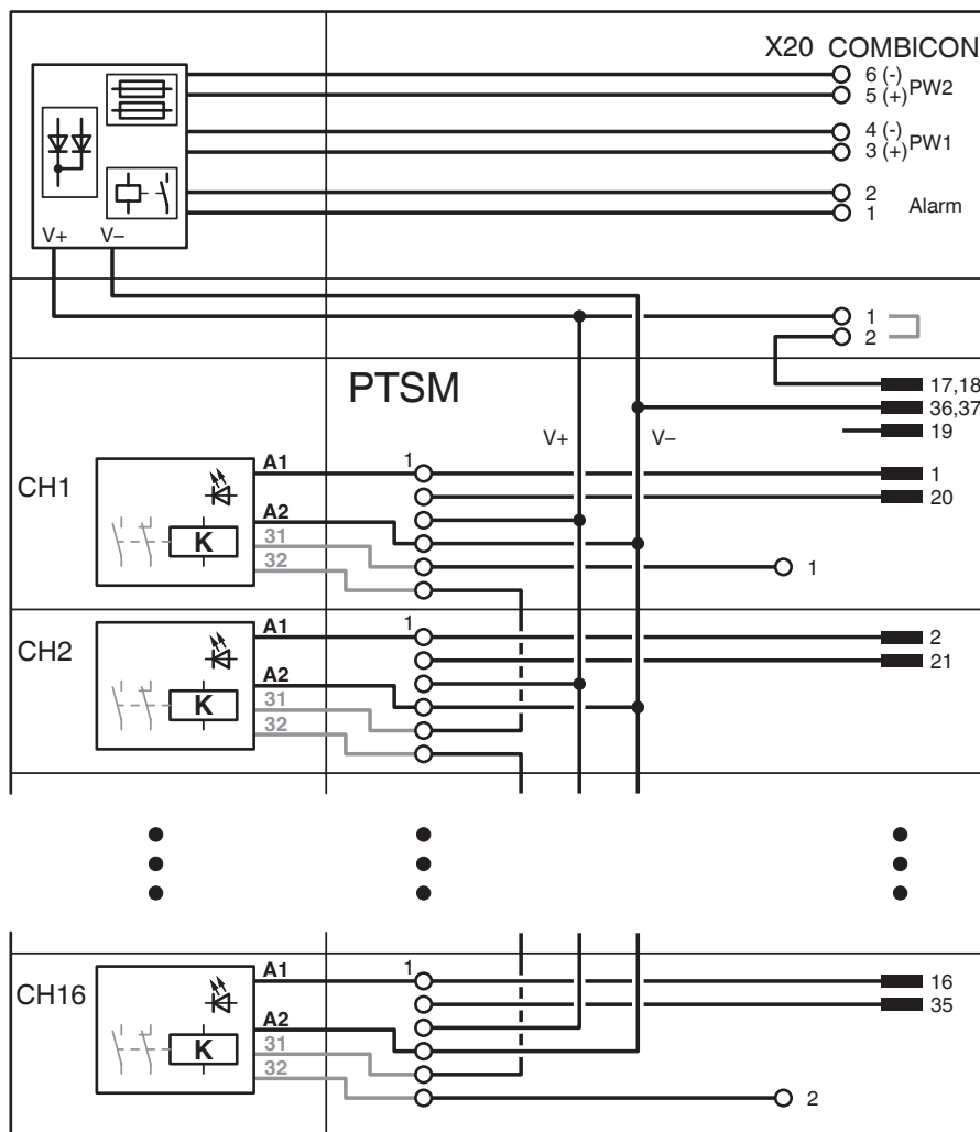
Esquema de conexiones TC-2D37SUB-DO16-ESD-AR-UNI
