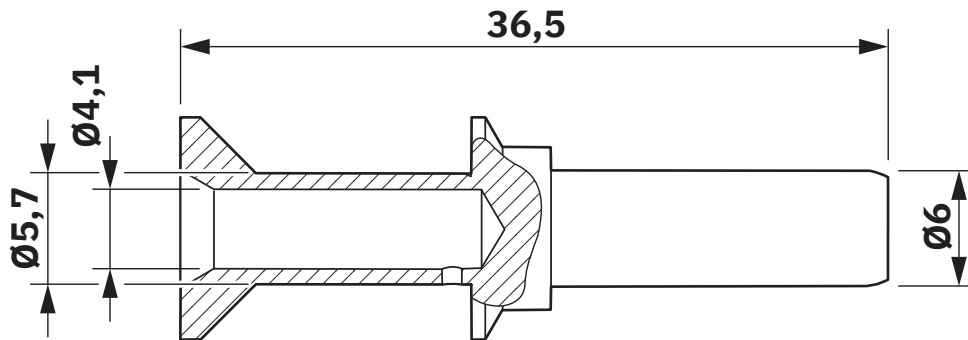
Maßzeichnung
