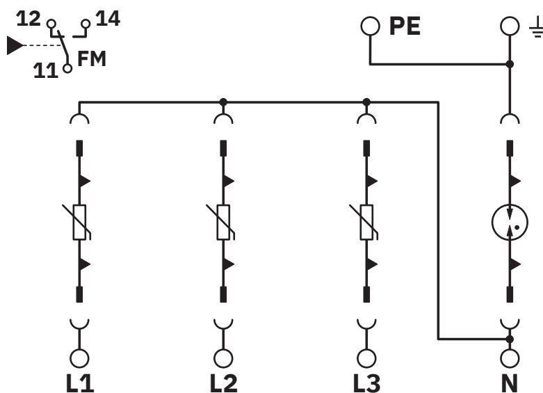
Diagrama eléctrico
