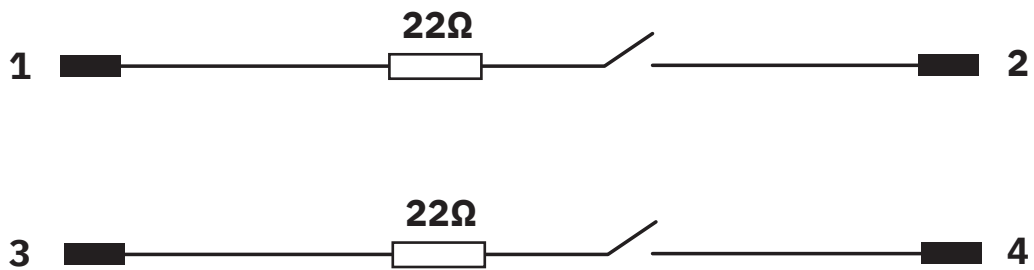
Schaltplan
