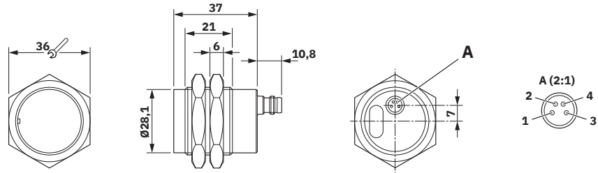
Maßzeichnung
