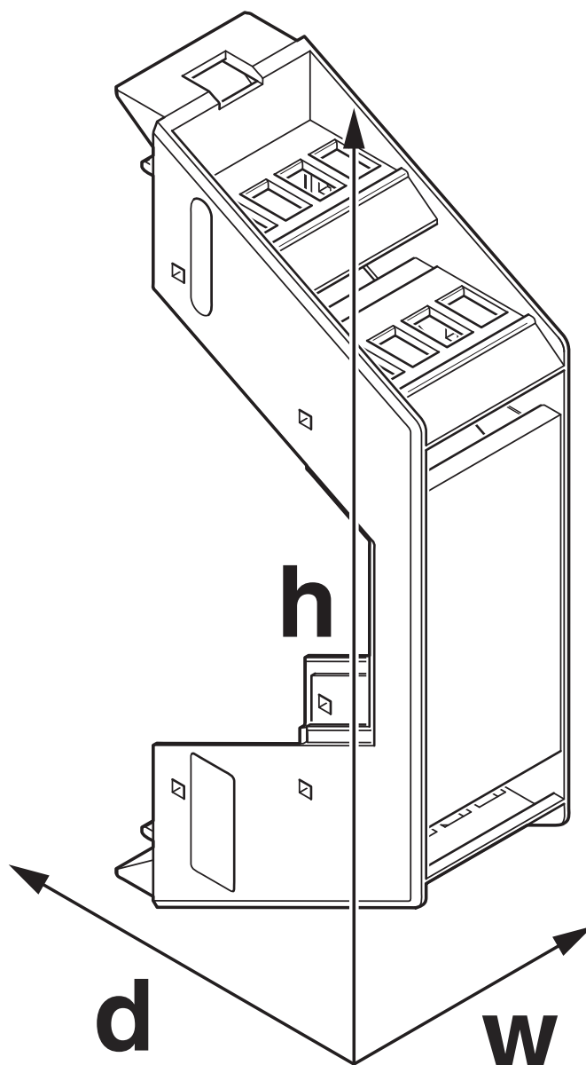
Dessin coté
