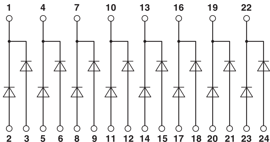
Schaltplan
