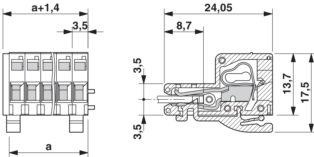
Dessin coté
