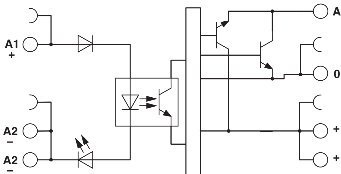
Diagrama eléctrico
