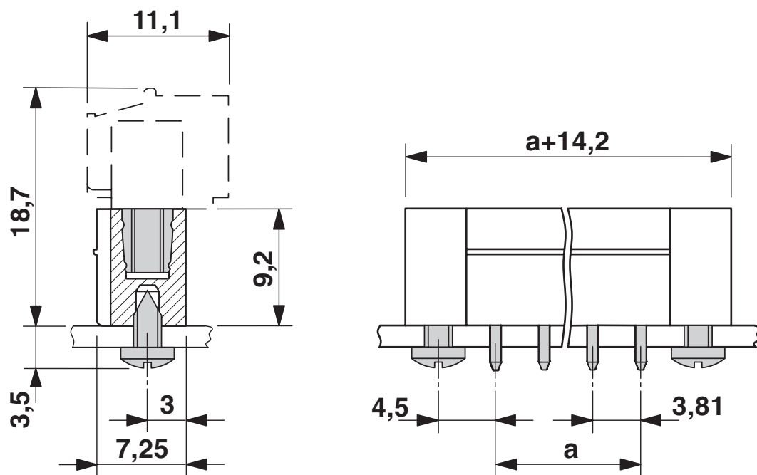
Maßzeichnung
