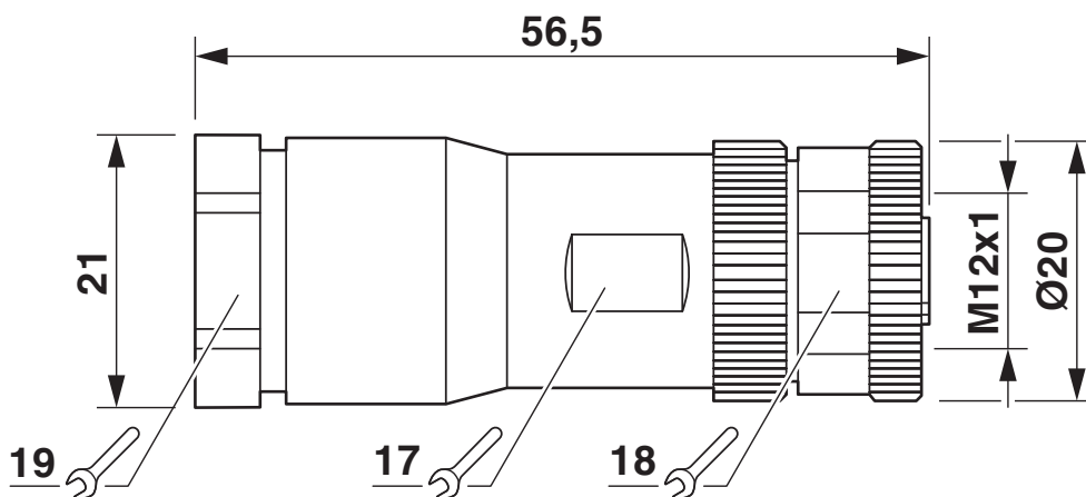
Maßzeichnung
