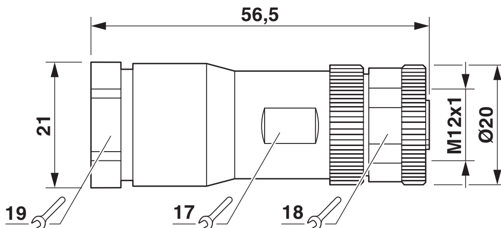
Dessin coté
