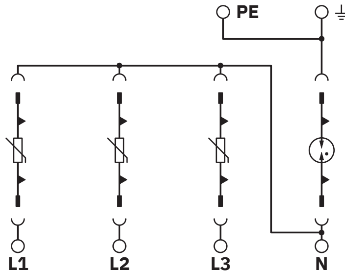
Schaltplan
