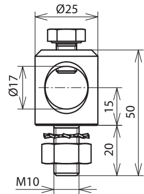
Maßbild BB16 GSM10 V2A
