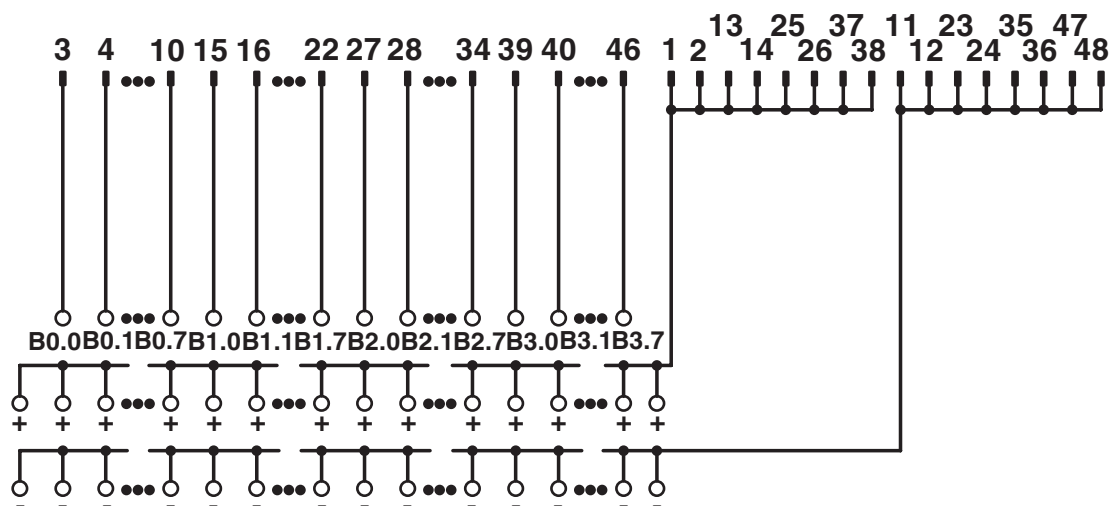
Diagrama eléctrico
