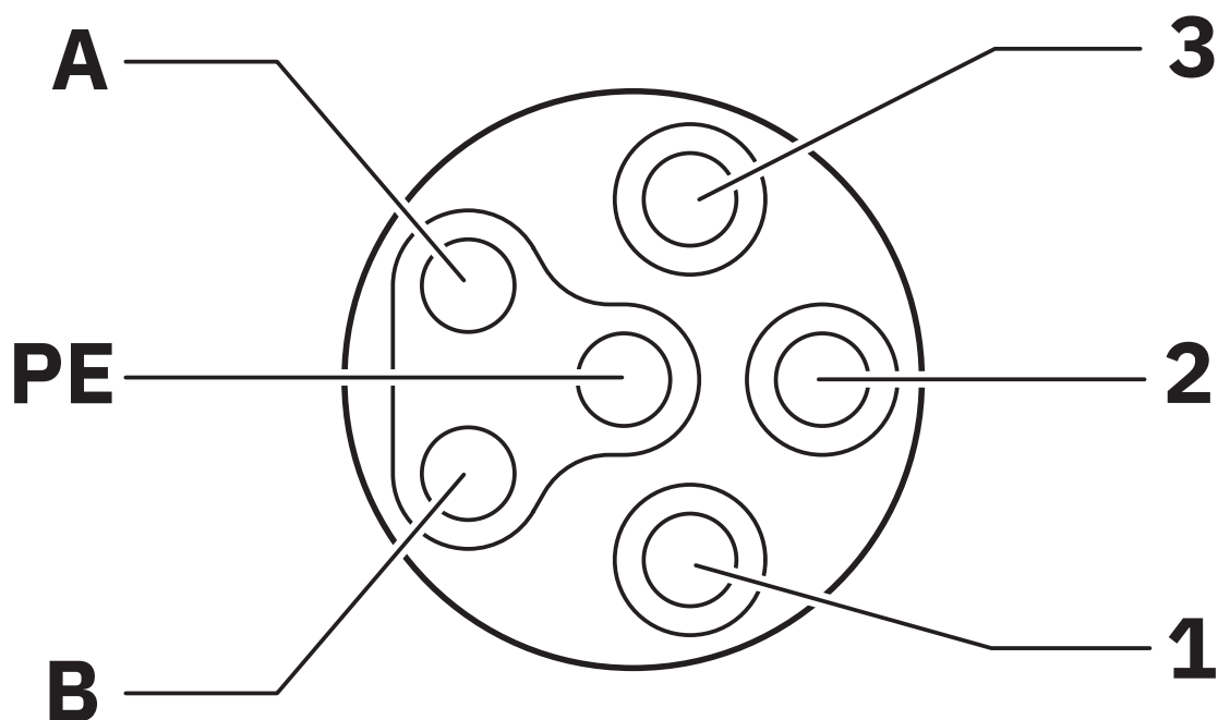
Esquema de polos de conector hembra S15 acodado a la derecha 90°, 6 polos, vista: lado de hembras
