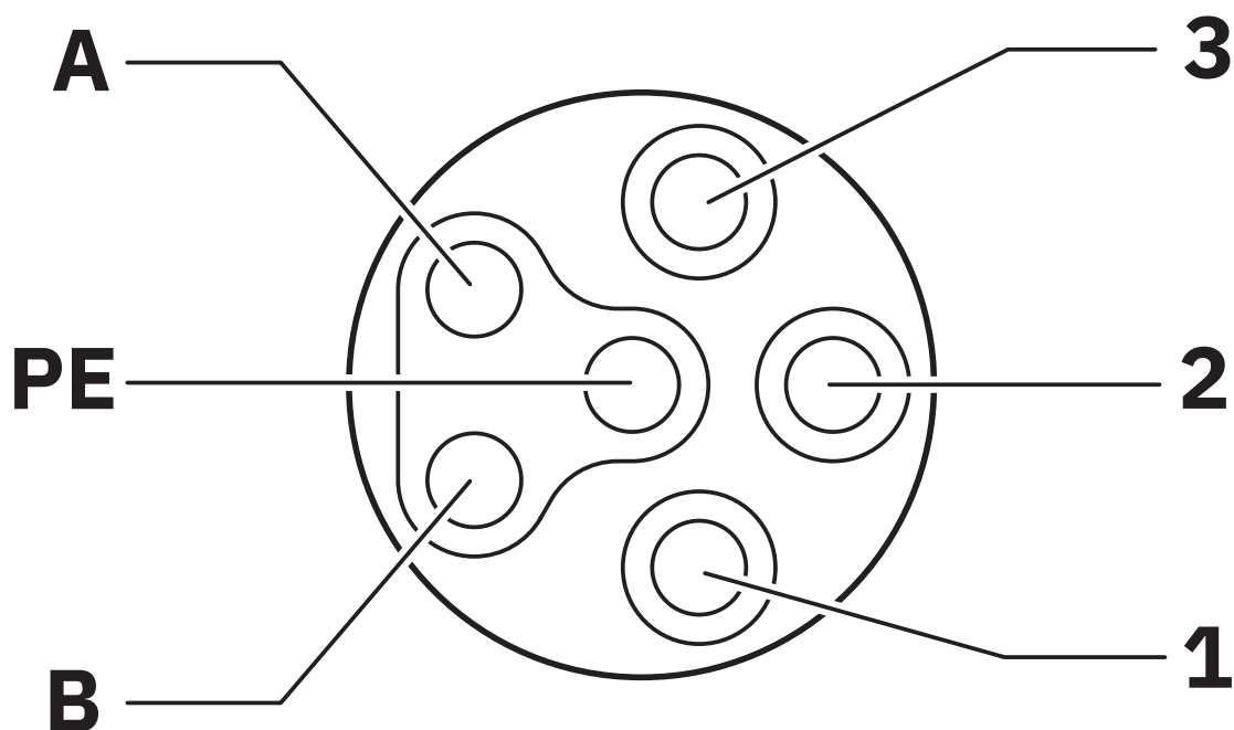
Schéma des pôles connecteur femelle S15 coudé vers la droite à 90°, 6 pôles, vue côté femelle
