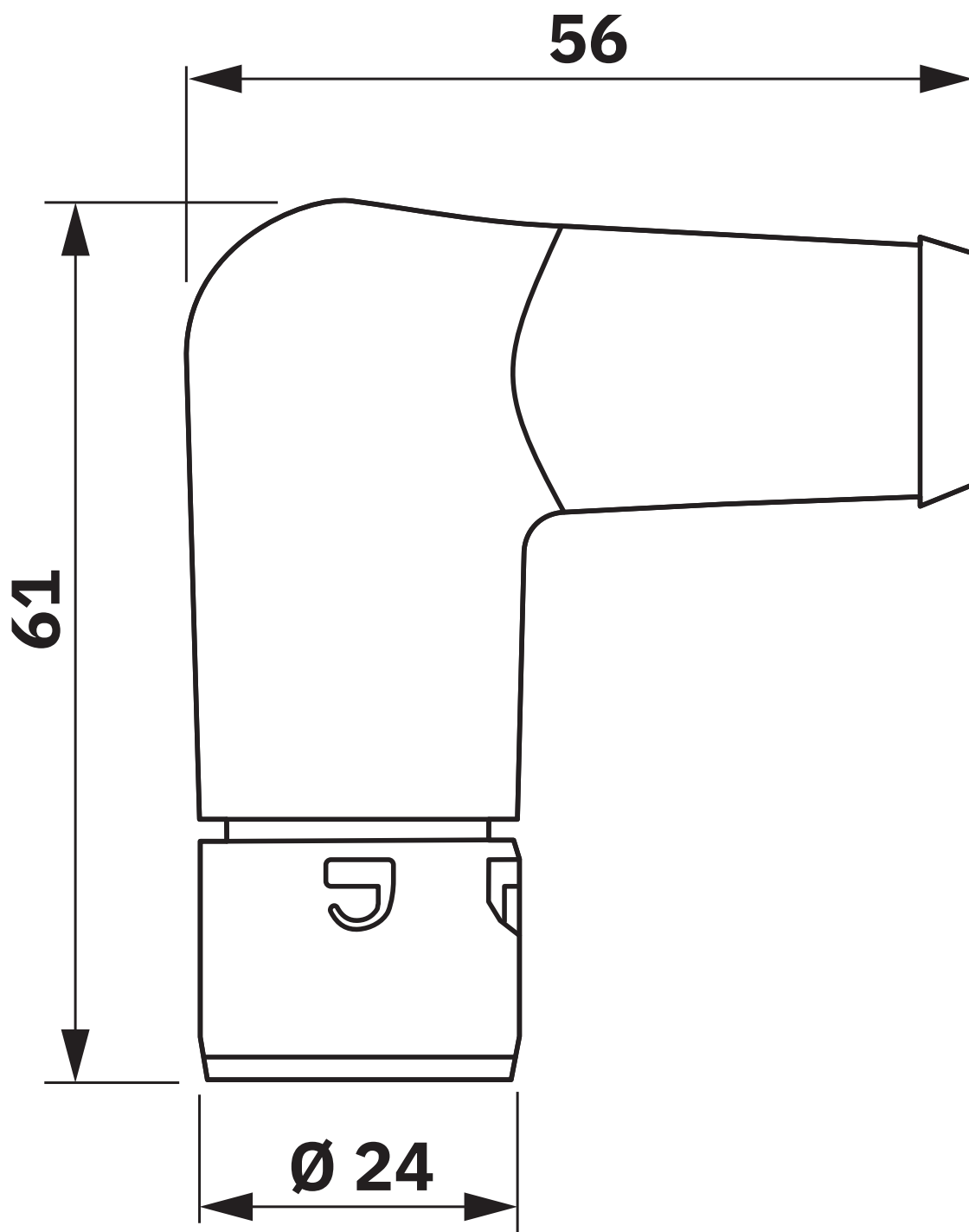
Connecteur femelle S15 coudé
