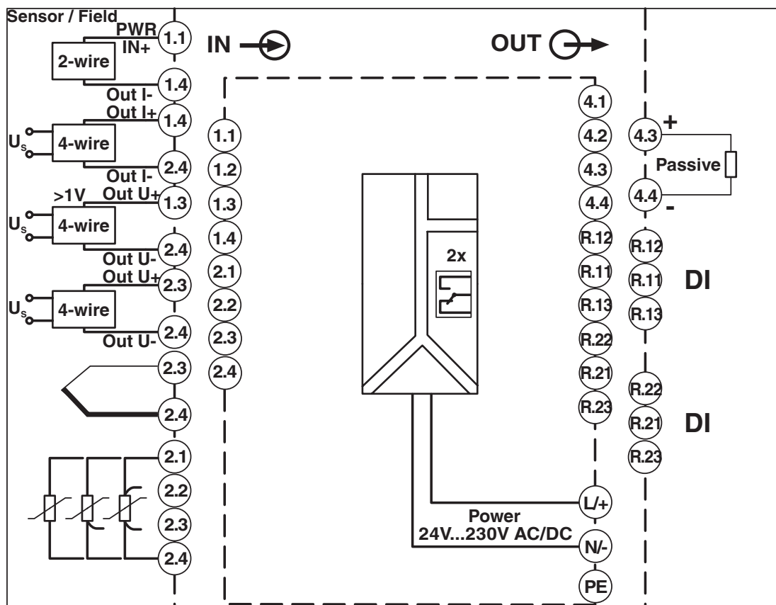
Blockschaltbild FA-MCR-D-TUI-UI-2REL-UP
