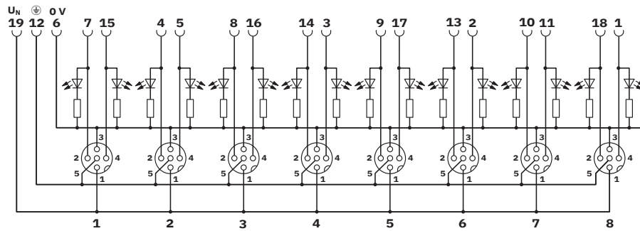
Diagrama eléctrico
