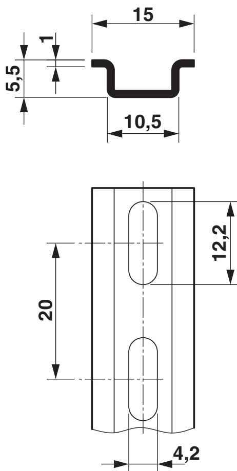
Dessin coté
