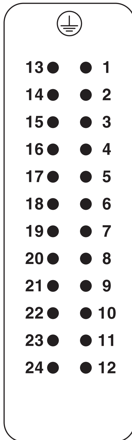
Schemazeichnung
