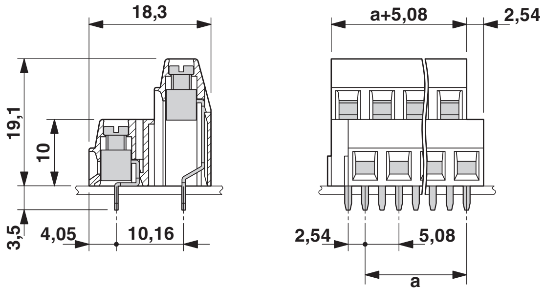
Maßzeichnung
