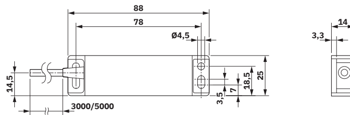
Maßzeichnung
