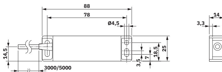
Esquema de dimensiones
