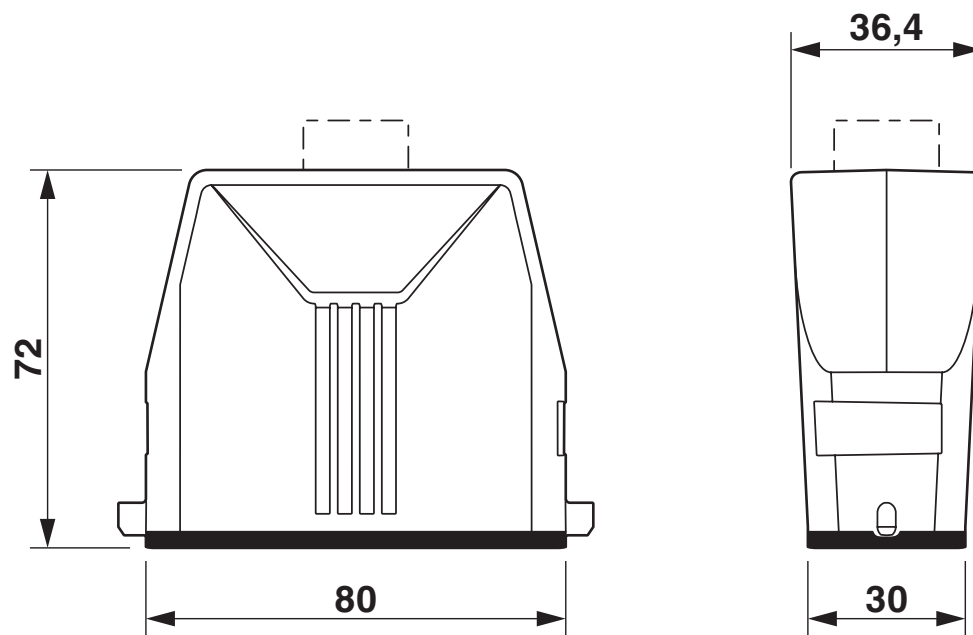
Maßzeichnung
