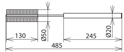
Maßbild RB 40 NS
