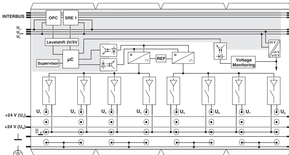
Schéma fonctionnel
