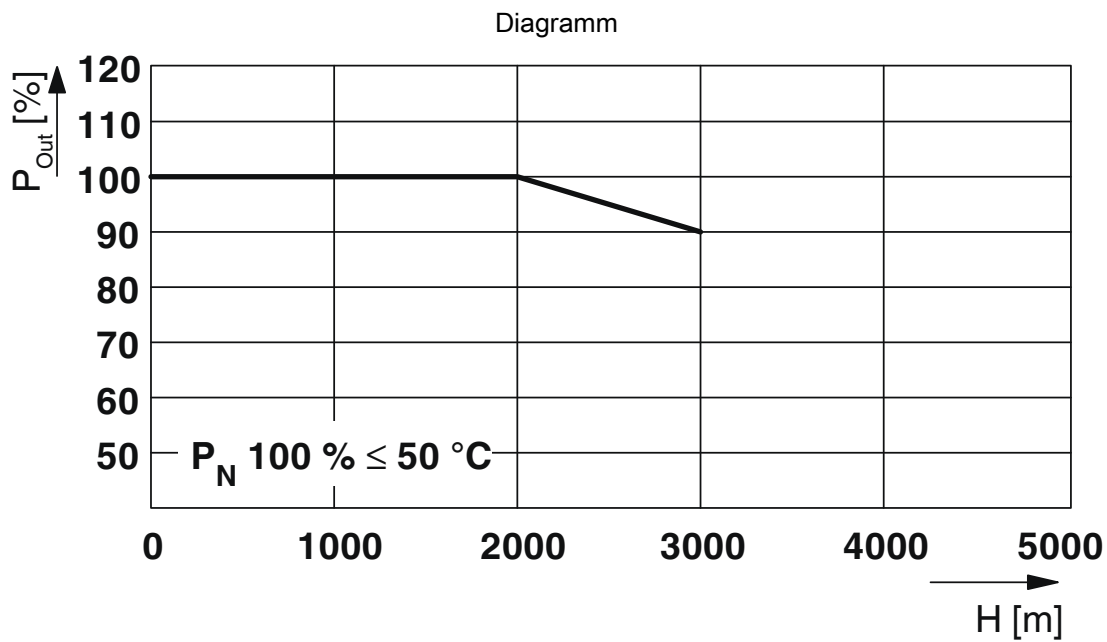
Ausgangsleistung/Aufstellhöhe
