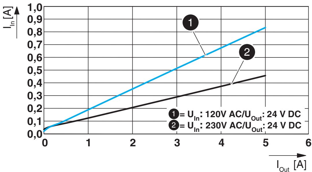
Eingangsstrom/Ausgangsstrom
