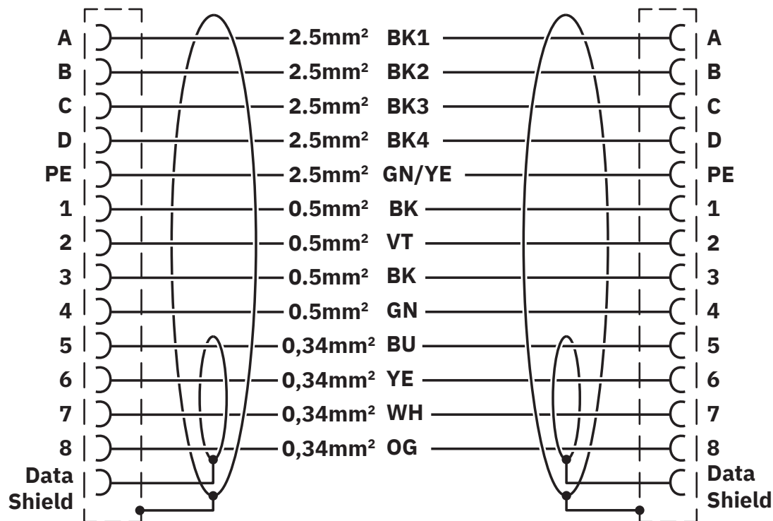
Schaltplan
