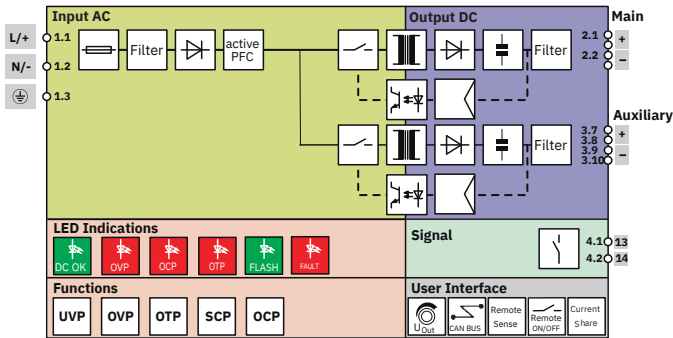
Schéma fonctionnel
