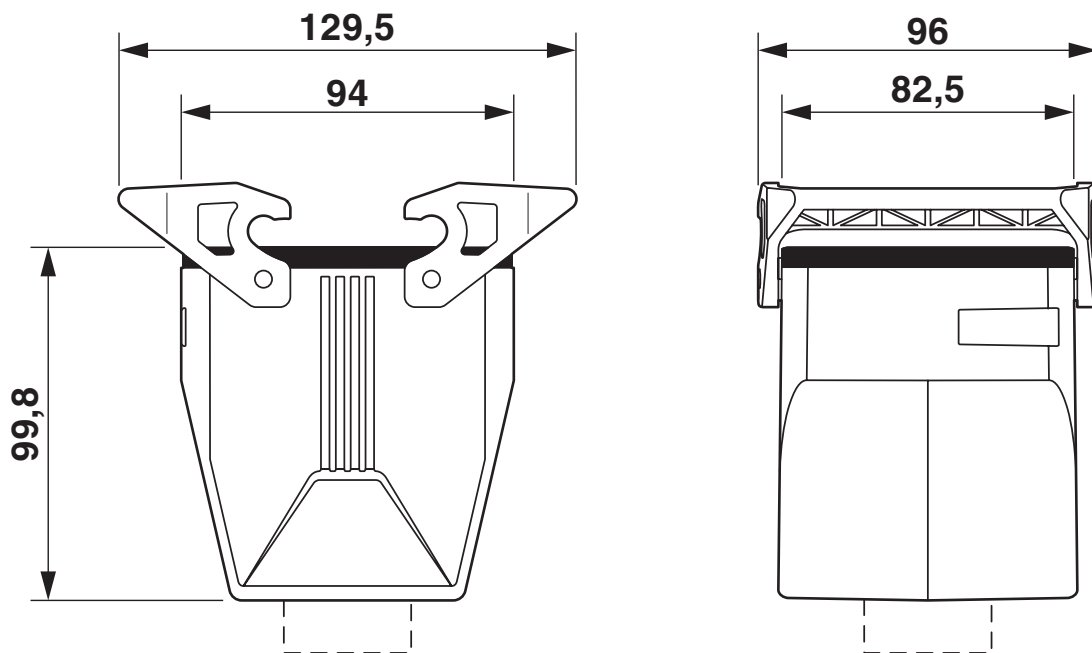
Maßzeichnung
