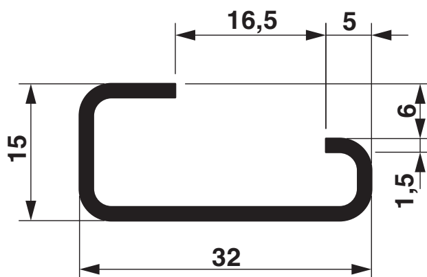
Maßzeichnung
