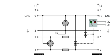
Complete module indirect grounding, with remote signalling Komplettmodul indirekte Erdung, mit Fernmeldung
