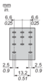
Stecker-Seitenansicht
