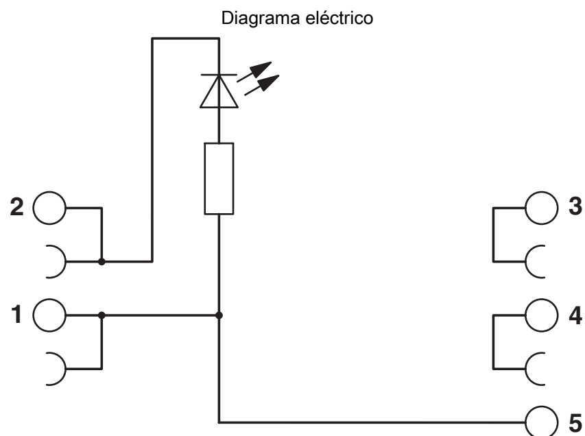
Esquema de conexiones PLC-VT/ACT/LA
