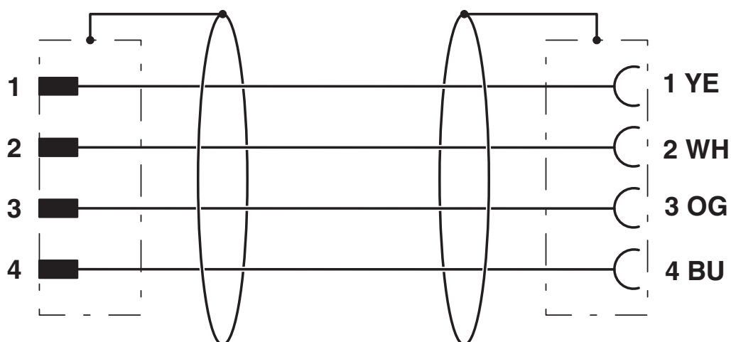
Disposition des contacts du connecteur M12 mâle et femelle
