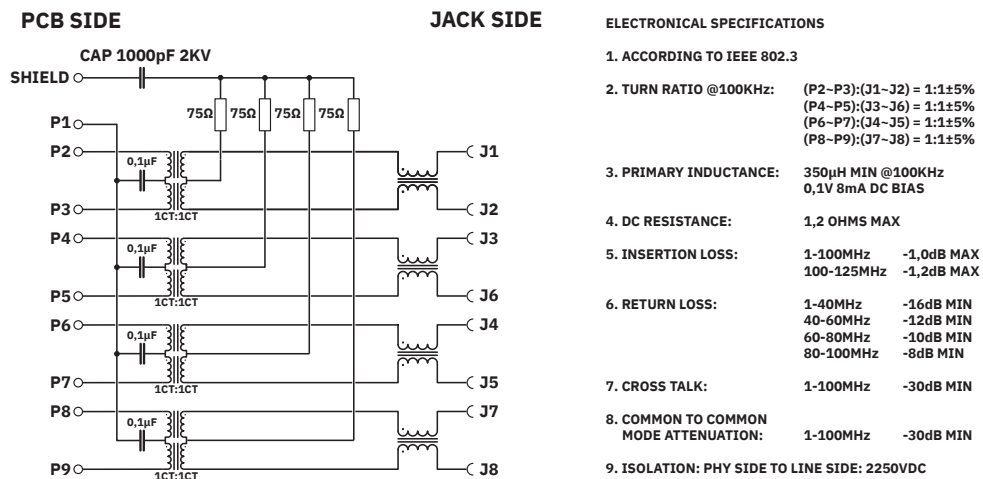
Schaltplan
