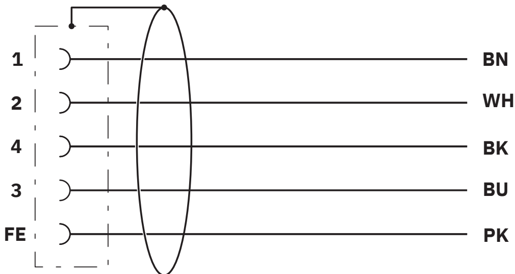
Kontaktbelegung der M12-Buchse
