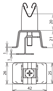
Maßbild LH ZG 8 H20 KB4.16 V2A
