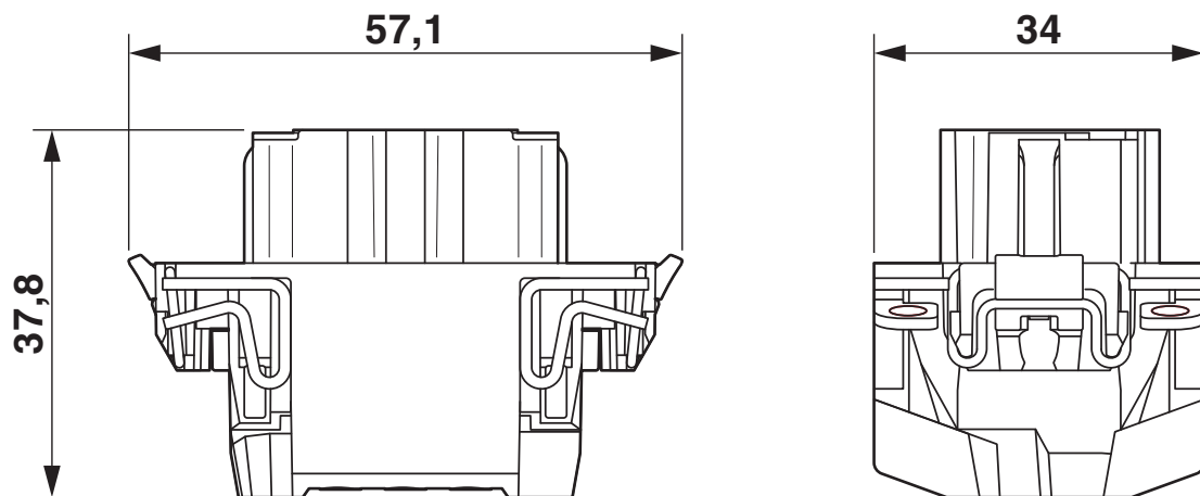
Maßzeichnung
