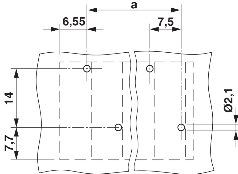
Bohrplan/Lötpadgeometrie
