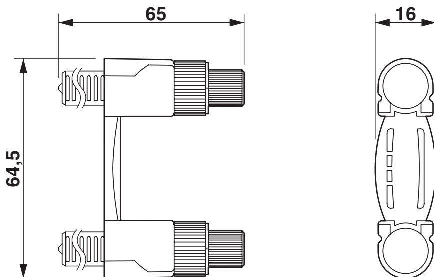
Dessin coté
