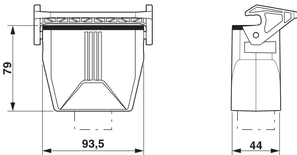
Maßzeichnung
