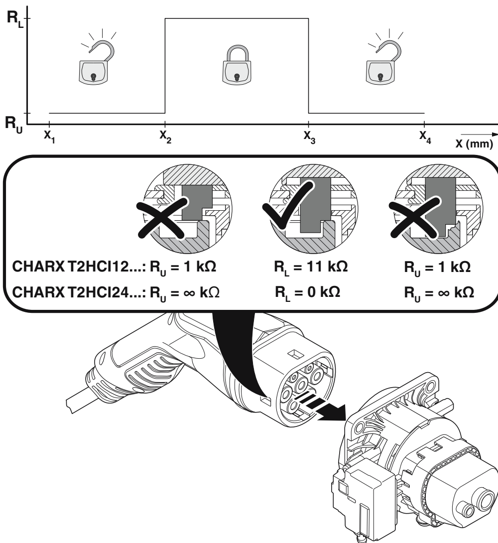
Dessin schématique
