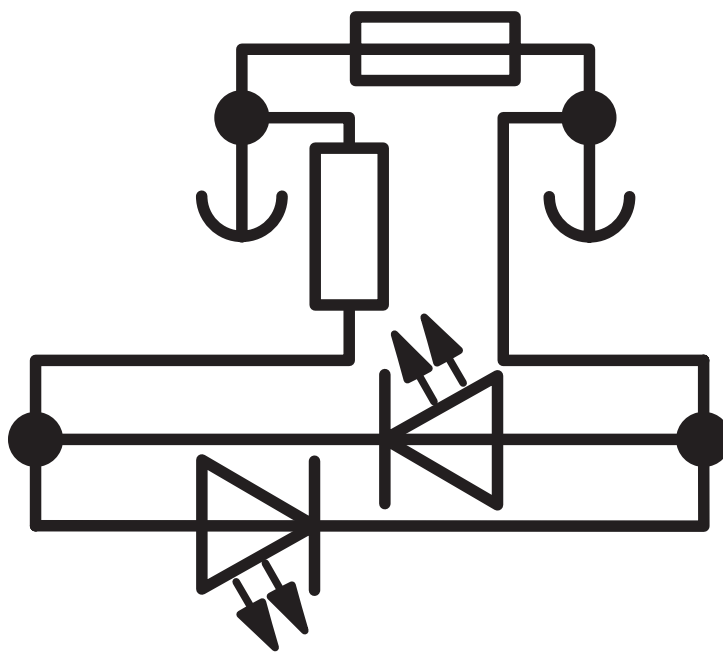
Diagrama eléctrico
