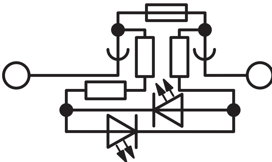
Diagrama eléctrico
