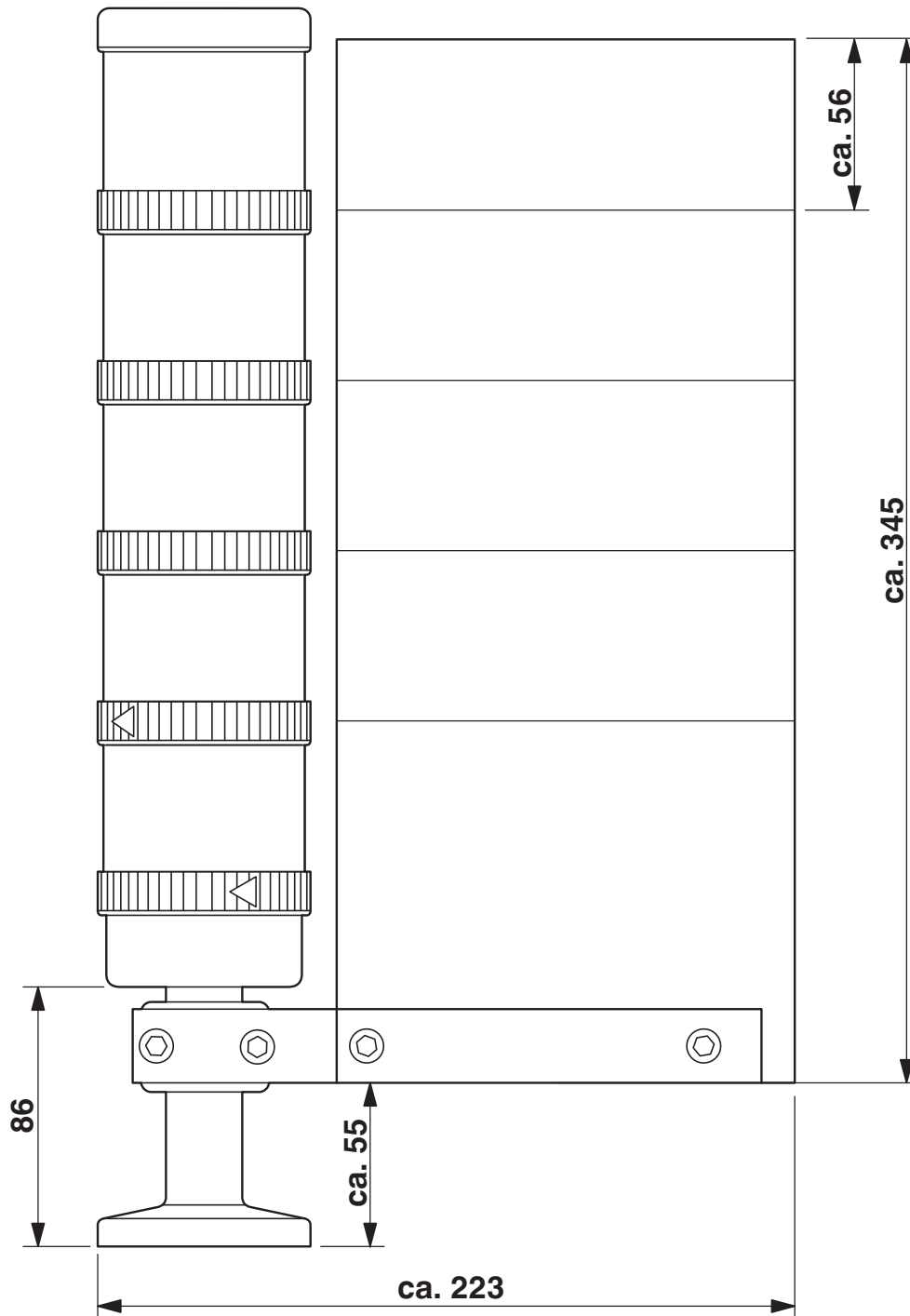
Maßzeichnung
