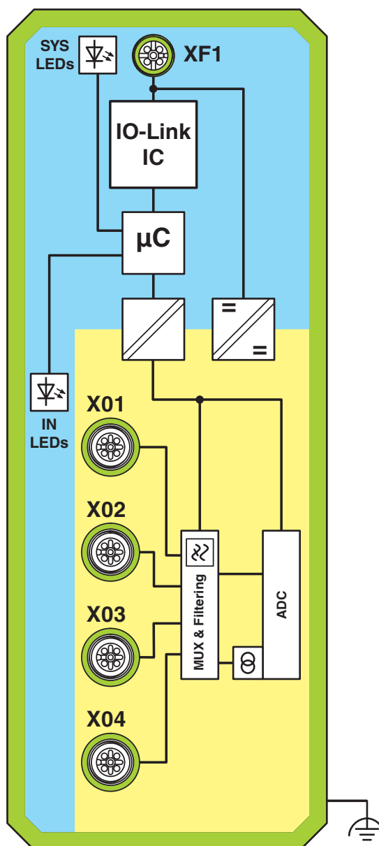
Schéma fonctionnel
