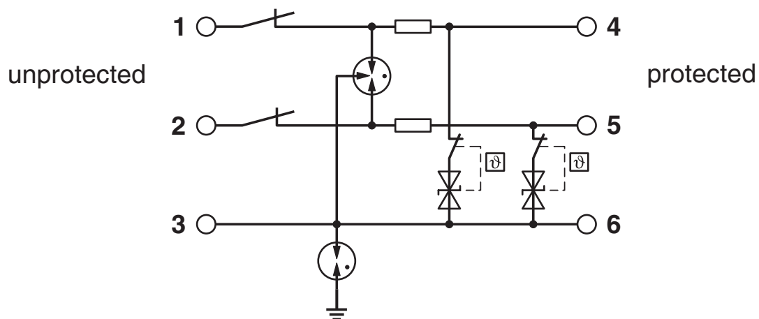
Diagrama eléctrico
