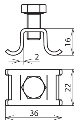
Maßbild SPK 14X0.3 V2A
