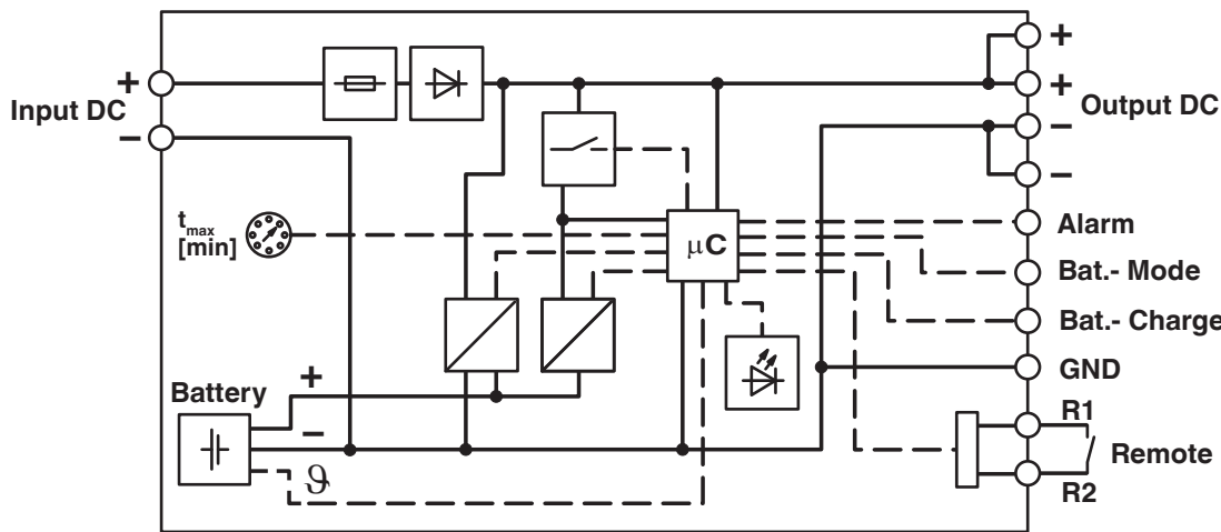
Schéma fonctionnel
